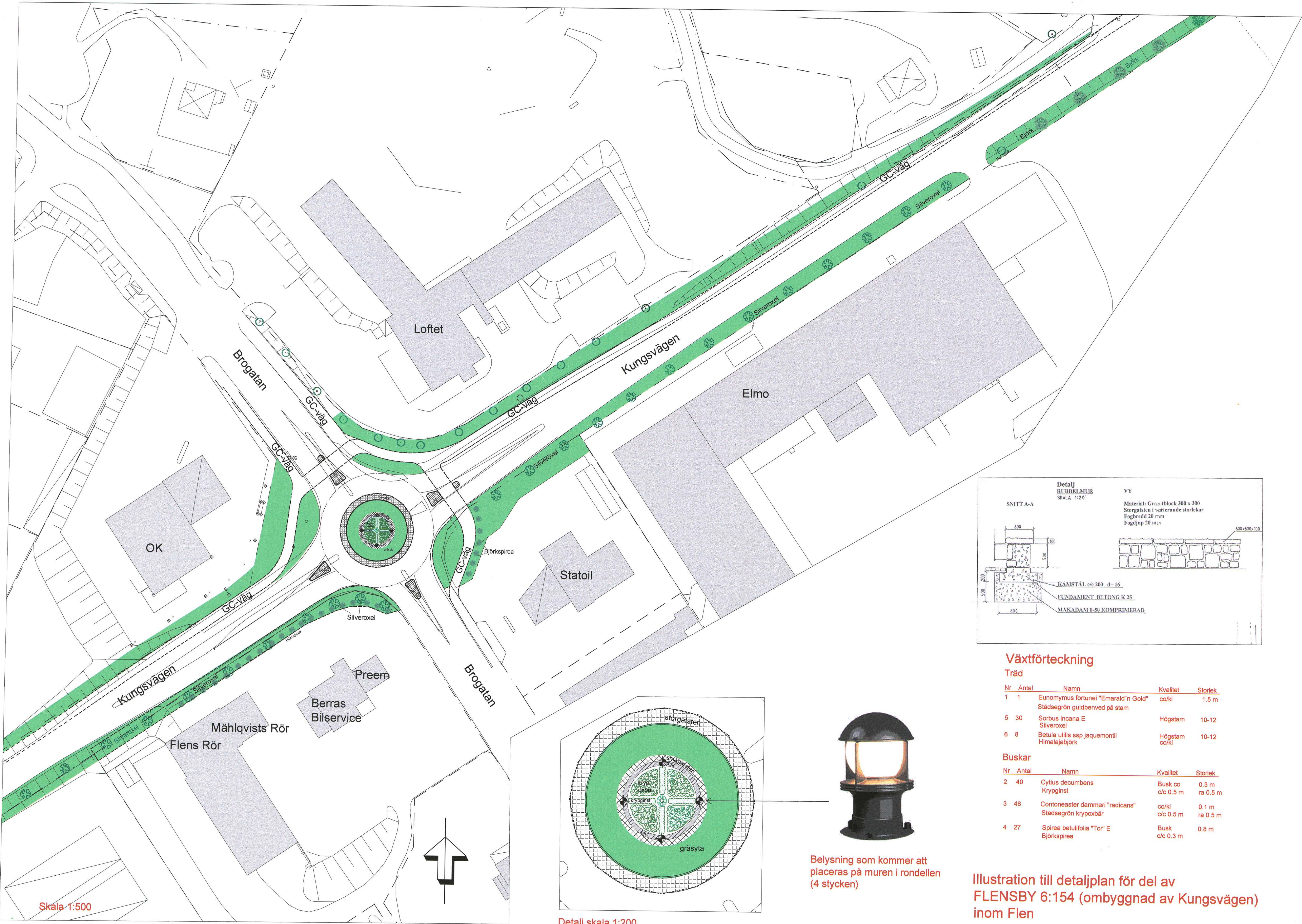
Detalj skala 1:200
